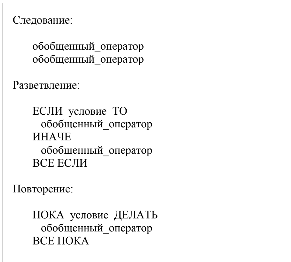
Рис. 8.2. Основные конструкции структурного программирования на псевдокоде.
