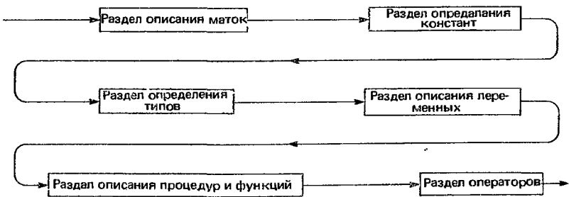
Р и с. 3.2. Синтаксическая диаграмма для Блока
