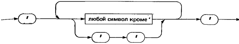
Р и с. 1.6. Синтаксическая диаграмма для Строки символов
