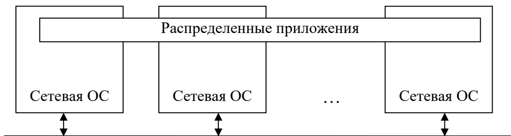
Рис. 75. Структура сетевой ОС.
