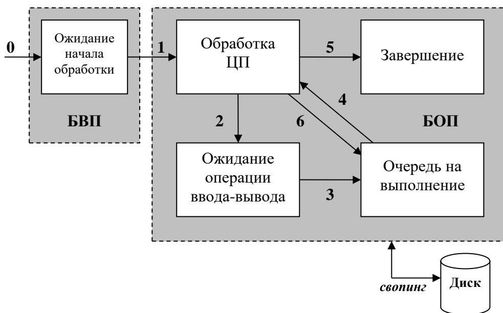
Рис. 80. Модель ОС с разделением времени (модификация). Заблокированный процесс может быть откачан (свопирован) на внешний носитель, а на освободившееся место может быть подкачен процесс с внешнего носителя, который был откачен ранее, либо взят новый.
