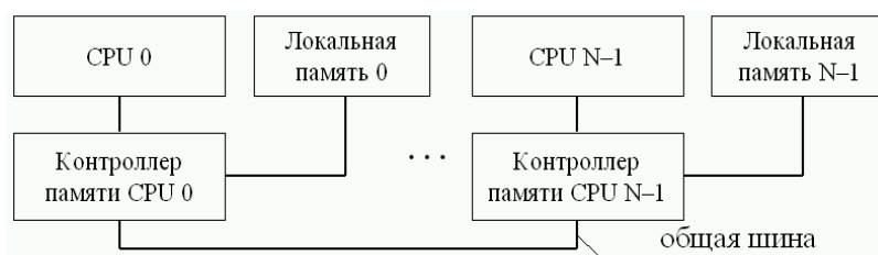
Рис. 61. Схема NUMA-системы
