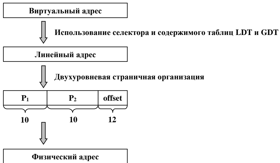
Рис. 144. Схема преобразования адресов.
