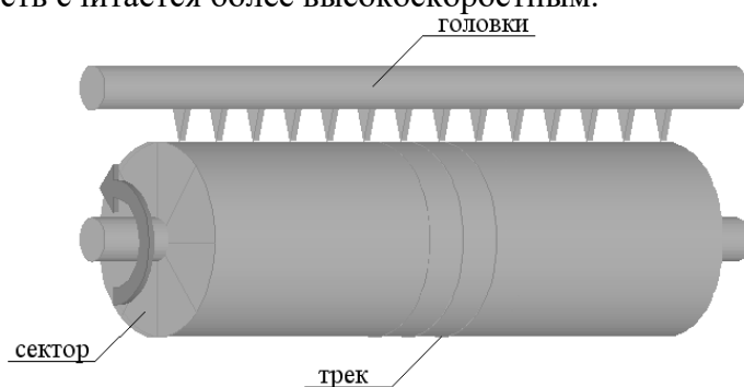
Рис. 37. Принцип устройства магнитного барабана.
