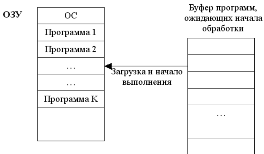
Рис. 47. Перемещаемость программы по ОЗУ.
