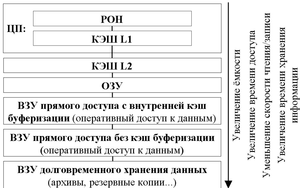
Рис. 43. Иерархия устройств хранения информации.
