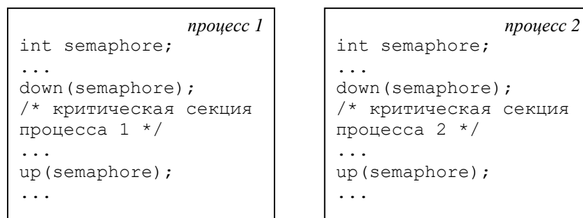
Рис. 93. Пример использования двоичного семафора для организации взаимного исключения.
