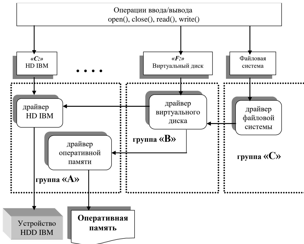
Рис. 6. Схема организации ввода-вывода в системе.
