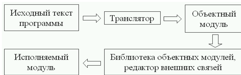
Рис. 46. Процесс получения исполняемого модуля программы.
