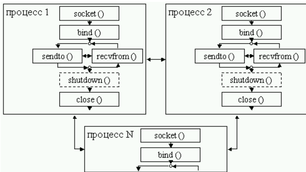
Рис. 102. Схема работы с сокетами без предварительного установления соединения.
