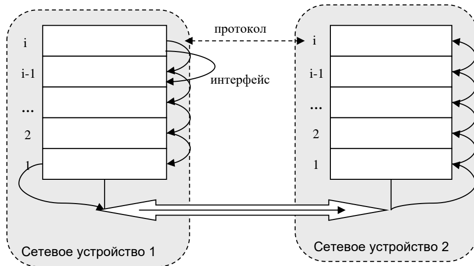
Рис. 67. Логическое взаимодействие сетевых устройств по i -ому протоколу.
