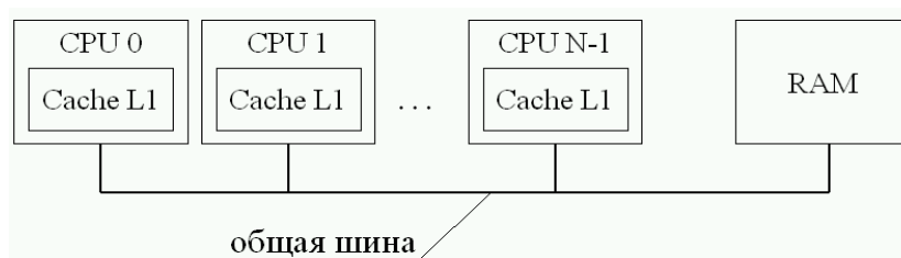
Рис. 60. Схема SMP-системы.
