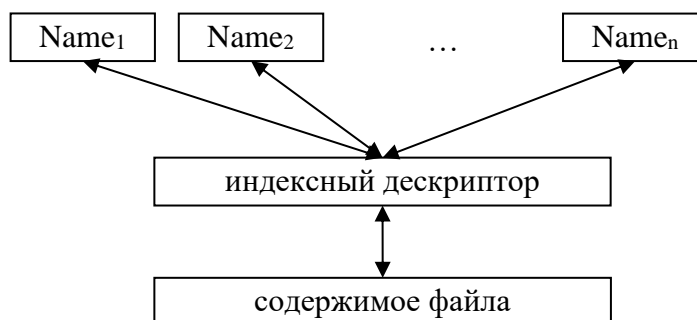
Рис. 122. Индексные дескрипторы.
