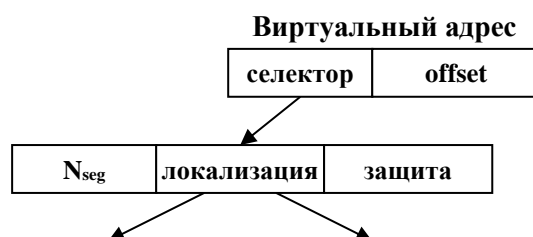
Рис. 143. Сегментно-страничное распределение. Упрощенная модель Intel.
